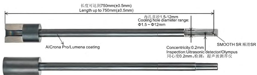
水孔镶件剖析图 Core Pins For HPDC/Jet Cooling
